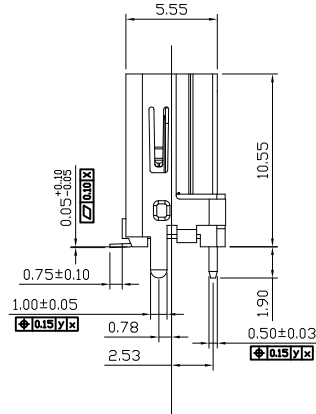
SECTION C 5:1
